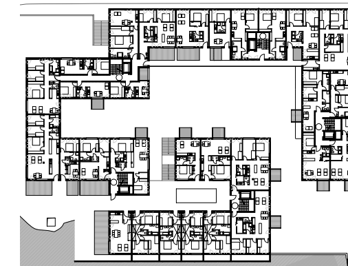
Ebene 3
