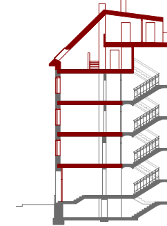
Schnitt
